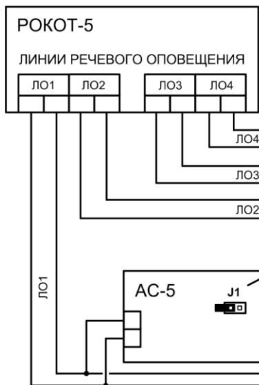
Рис.А4 Схема подключения «АС-5» к линиям оповещения «РОКОТ-5 ПУО-100»
