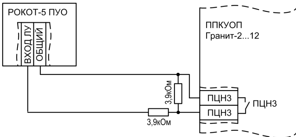
Рис. А2 Схема подключения ПУО к ППКУОП «Гранит-2,-3,-4,-5,-8,-12,-16,-20,-24»
